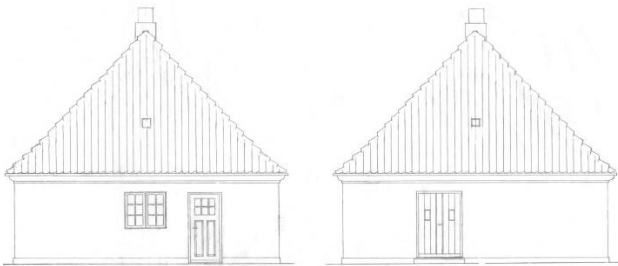
Øst- og vestgavle - før restaurering
