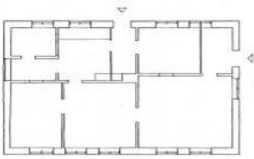
Plan af Spindeskolen - før restaurering
